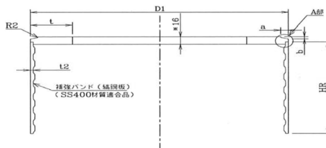
R 型 (溝鋼板方式) 頭部・継手金具
